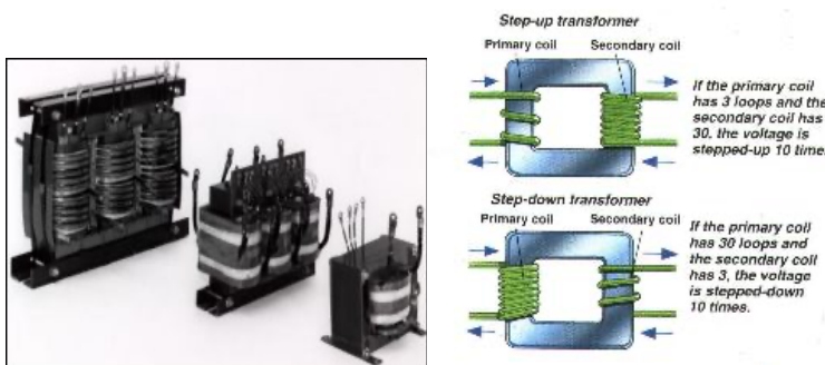
Transformadores y detalles de un transformador
