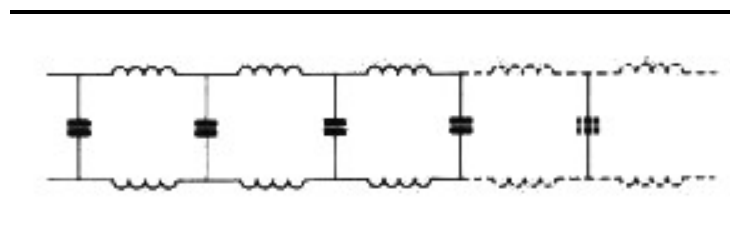
Circuito equivalente de una línea de transmisión
