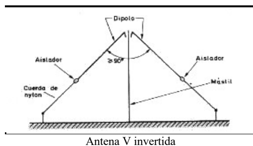
Antena V invertida
