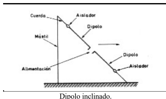
Dipolo inclinado.
